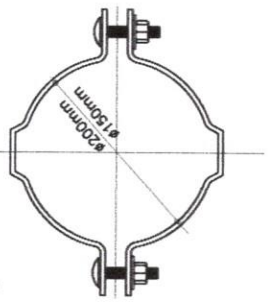
DET. CINTA (ABRACAÇADEIRA) ESCALA-1/6.25
